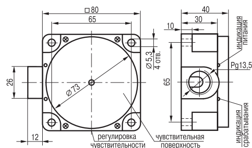
Габаритный чертеж
